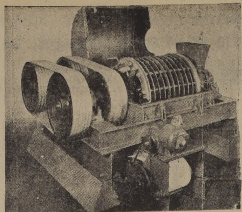
Una de las modernas máquinas que se emplea en los nuevos procedimientos de molienda integral, en Estados Unidos
