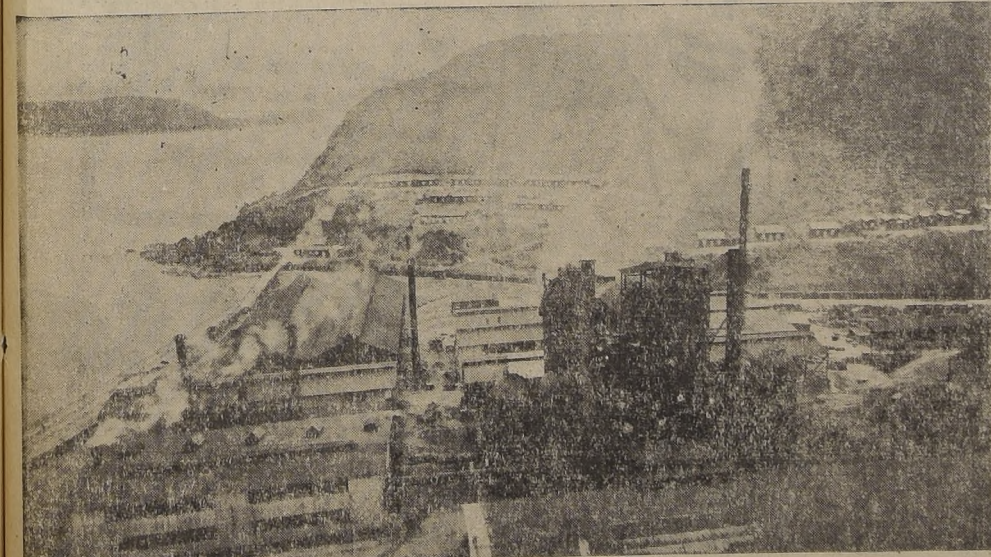
En esta fotografía figura en primer término, a la izquierda, la Central de Fuerza de Corral; en seguida, la Maestranza y los Hornos de Aciería. — Al centro, los Altos Hornos, complementados con otras instalaciones. — Al fondo, una parte de la población Obrera de la Compañía
