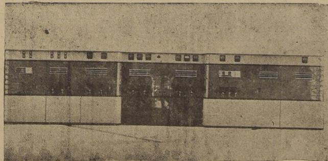
UNO DE LOS PODEROSOS TRANSMISORES CONSTRUIDOS ESPECIALMENTE PARA LA CORPORACION CHILENA DE BROADCASTING POR LA R. C. A.
