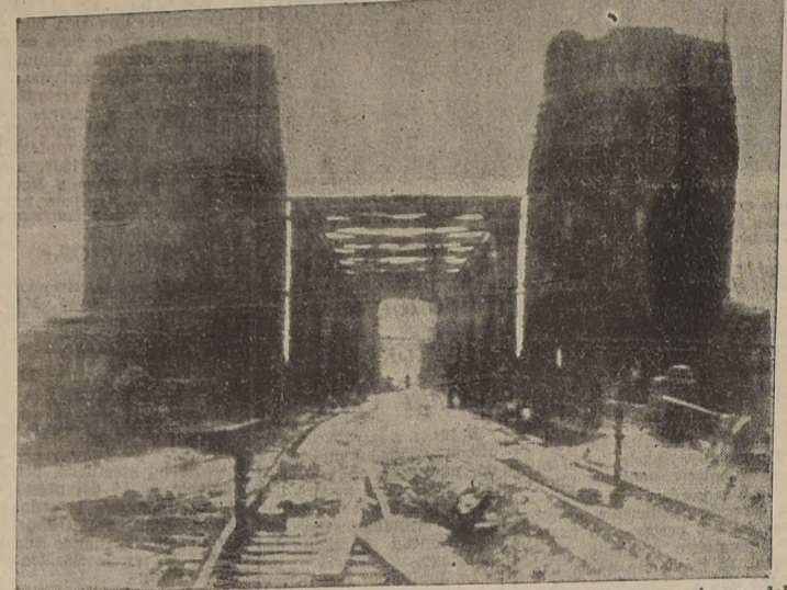
Este es el puente de Remagen sobre el Rhin, cruzado por las fuerzas norteamericanas del general Courtney Hodges, las que ya han establecido una cabecera de puente en la oriental del río, dando comienzo así al capítulo final de la guerra en Europa.
