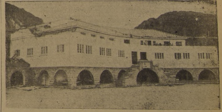
Edificio principal de cantera y hormigón para pabellón de cabinas y un restaurante con todos sus anexos, donde antes existían vetustas armazones de madera sobre una puntilla del cerro
