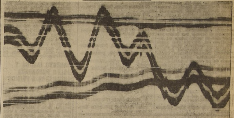
Registros de los Inclínógrafos del Observatorio del Salto; movimientos imperceptibles de la corteza terrestre, registrados automáticamente por procedimientos óptico-fotográficos, con amplificación de CIEN MIL VECES, del orden del microscopio electrónico. Este nuevo método de estudio no era conocido hasta ahora.
