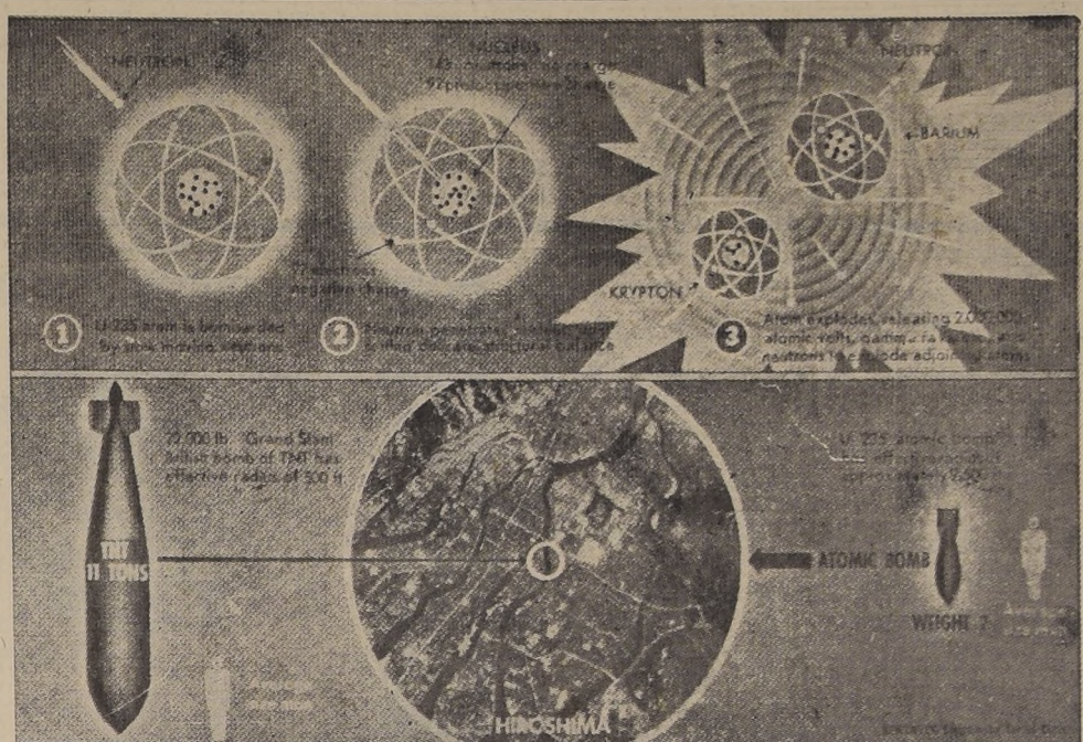
El presente diagrama proporciona una explicación elemental y aproximada del proceso de la desintegración del átomo, punto inicial de las investigaciones y descubrimientos que han conducido a la invención de la bomba atómica. La figura No. 1 señala el momento en que un átomo de uranio inestable es bombardeado por neutrones de movimiento lento. (Los átomos de uranio están compuestos por un núcleo central formado por 143 neutrones cargados de electricidad negativa y por 92 protones positivos de carga positiva, y por 92 electrones de carga negativa). El No. 2 indica el momento en que los neutrones penetran en el núcleo destruyendo el delicado equilibrio que mantiene la estructura del átomo. Y finalmente, el No. 3, corresponde a la explosión del átomo. Al estallar el átomo de uranio isotópico o inestable (U 235) se desintegra produciendo bario y kriptón. Como el monto de estos cuerpos es inferior al del uranio, la diferencia surge como energía explosiva. Esta energía ha sido calculada en 2.000.000 de voltios atómicos. La explosión produce también rayos gamma, etc., y neutrones que contribuyen a hacer estallar a los otros átomos adyacentes.
