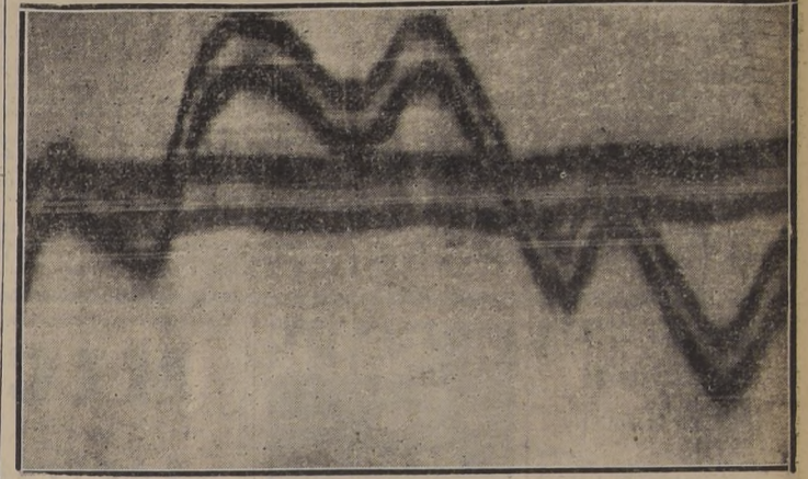
En los Inclinógrafos del Observatorio del Salto se vienen registrando desde marzo "ondas Bradisísmicas" de extraordinaria intensidad, que precedieron al Maremoto del Pacífico
