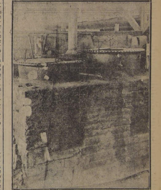
Horno para el cocimiento de aceites para pinturas
