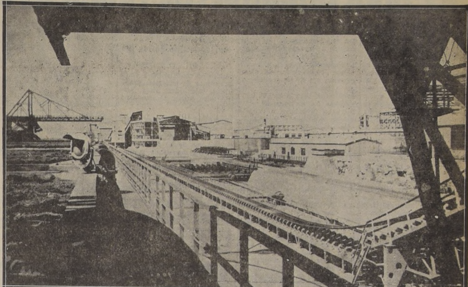
Vista parcial de "Pedro de Valdivia" en que aparece la correa transportadora que lleva el caliche de los molinos a los estanques de lixiviación
