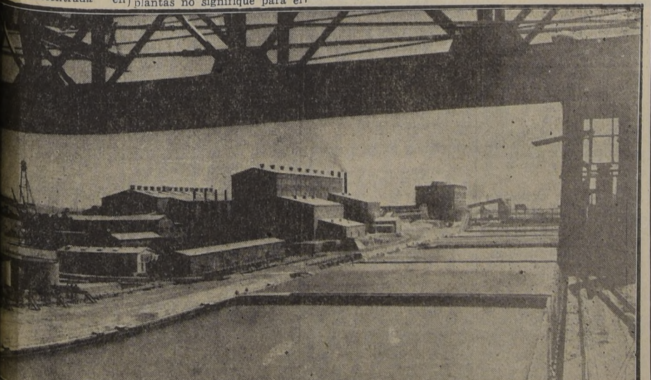
Vista parcial de "Pedro de Valdivia" en que se ven, en primer plano, los estanques de lixiviación. En estos estanques el caliche se separa el salitre o nitrato de sodio que se extrae de los estanques en forma líquida
