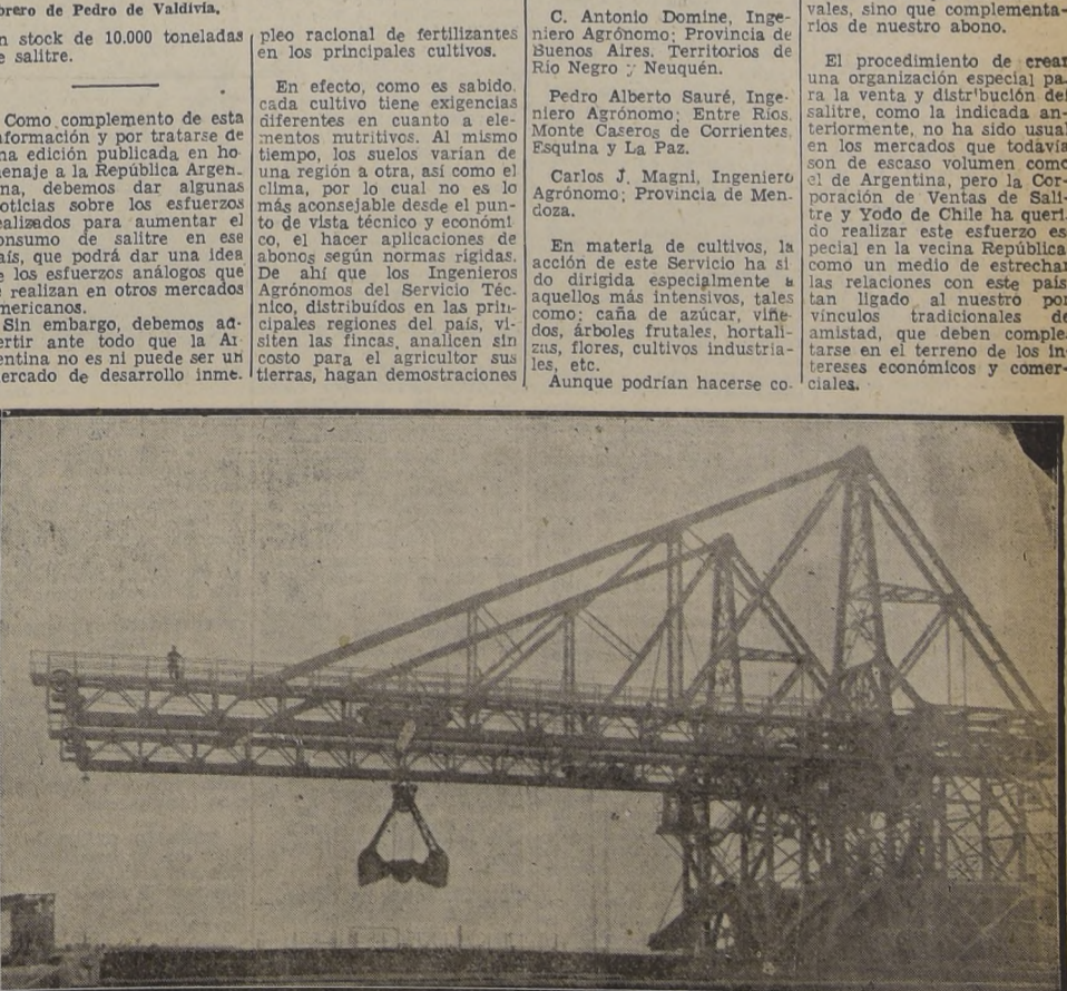
Puente de descarga de riplo de la Oficina "María Elena". Separado el salitre y extraído por cañerías de los estanques, quedan estos riplos que a su vez son extraídos mediante el empleo de este enorme puente mecánico
