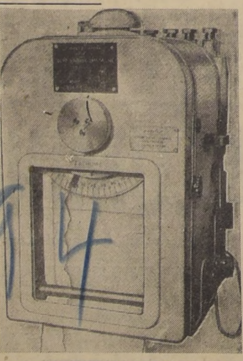
REGISTRADOR DEL ECOSONDA HUGHES M. XX
