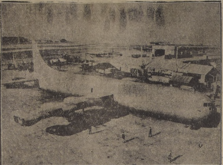
El próximo mes de abril será probado por primera vez por la Fuerzas Aéreas del Ejército este gigante avión que puede transportar 400 pasajeros o 50.000 kilogramos de carga a una distancia de 12.500 kilómetros. Este nuevo avión, el XC-99, tiene una amplitud de alas de 80 metros, y un largo de 60. El XC-99, que tiene dos cubiertas anexas en esta foto en los patios de la Consolidated Vultee Aircraft Company. — (FOTO ACME)
