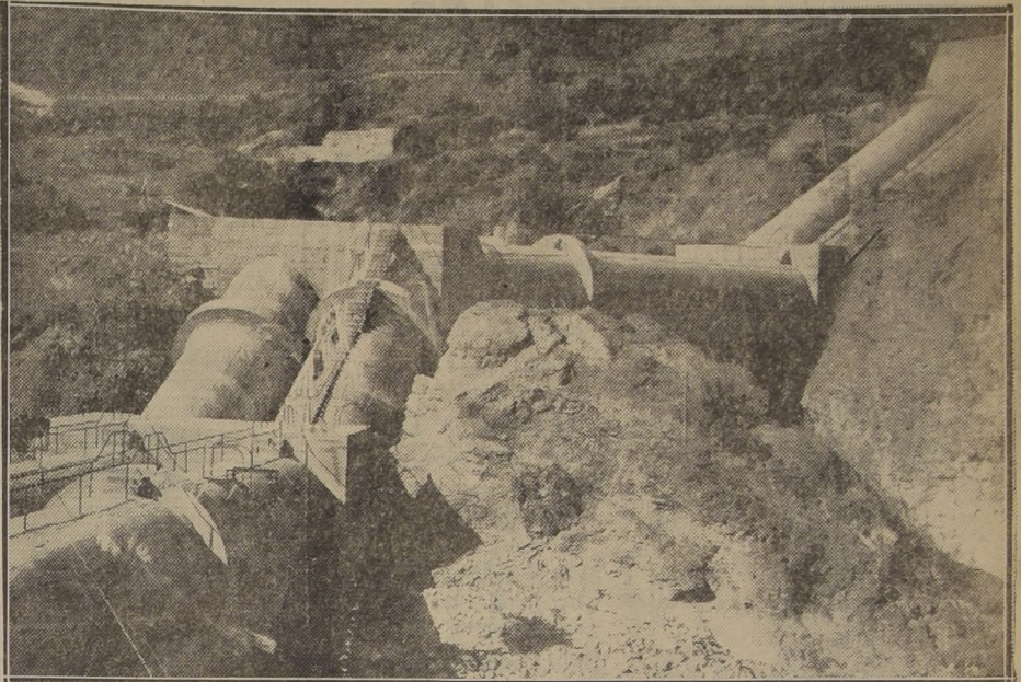
Aspecto del "Sifón del Gringo", gigantesca obra de ingeniería, que induce las aguas canalizadas de la ribera sur a la ribera norte del río Cachapoal.— En su género, este sifón es, sin duda, una de las obras de mayor importancia técnica en Sud América.
