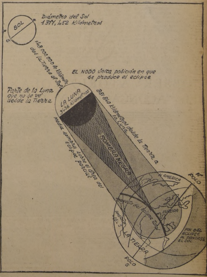
Diagrama del eclipse total de sol ocurrido el 28 de mayo de 1900, que fué muy similar al que se registrará pasado mañana.
