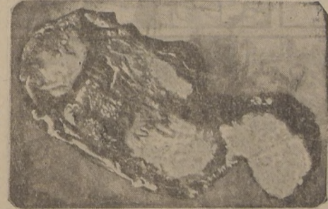
La Bacteria de Tuberculosis Bovina, ampliada a 125.000 veces, por un Microscopio Electrónico.
