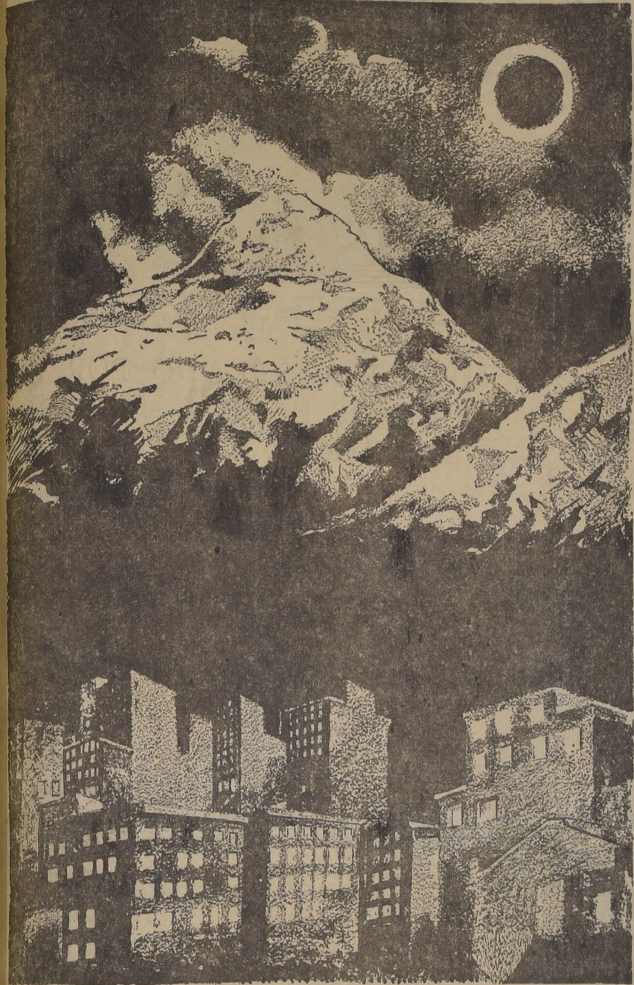
Desde el noveno piso de "LA NACION", nuestro dibujante Enrique Mosella da una visión de lo que será el eclipse de martes en su fase culminante.
