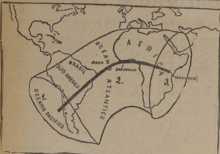
Trayectoria del eclipse total de sol del próximo martes 20 de mayo, según los cálculos del Observatorio del Salto; en la Zona 1, pleno día comienza a la salida del Sol; en la Zona 2, ocurre en pleno día y en la Zona 3, termina a la puesta del Sol. La sombra del eclipse total corre desde el centro de Chile hasta el África.
