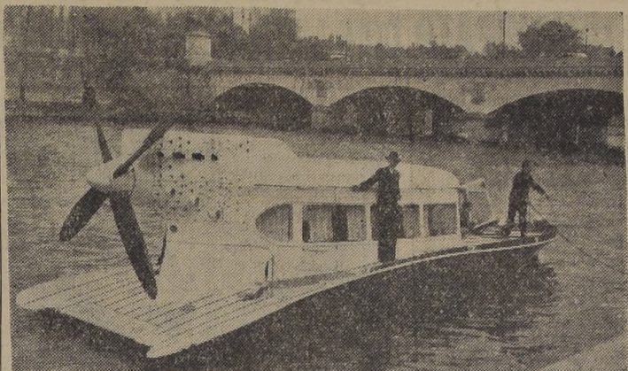
PARIS.—El hidrodeslizador "Arc en Ciel", el más grande aparato de su tipo en el mundo, en los momentos en que atraca en aguas del Sena después de su llegada a París. Esta embarcación marítima y aérea fue construida por A. A. Couzinet, en Brasil; puede lograr una velocidad de 93 kilómetros por hora y tiene capacidad para 22 pasajeros, fuera de sus dos hombres de tripulación. Couzinet lo bautizó con el nombre de "Arc en Ciel" ("Arcoiris"), en recuerdo del avión que construyó para el aviador francés Jean Mermoz, en 1932. — (Foto ACME).
