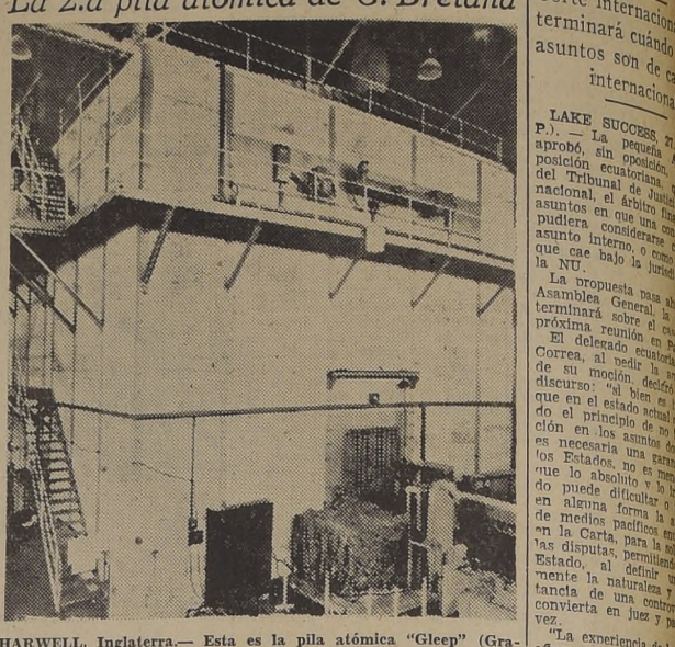
HARWELL, Inglaterra.— Esta es la pila atómica «Gleep» (Graphite Low Energy Pile: Pila de Granito de Baja Energía). En las esquinas más bajas están las cámaras que contienen el gas de trituro de boro, empleado para medir la intensidad de los neutrones en la pila, y, por consiguiente, para controlar el nivel de poder a que la pila es operada. La cara «de control» está a la izquierda, y a la derecha se hallan algunos instrumentos destinados a la preservación de la salud del personal.—(Foto ACME)
