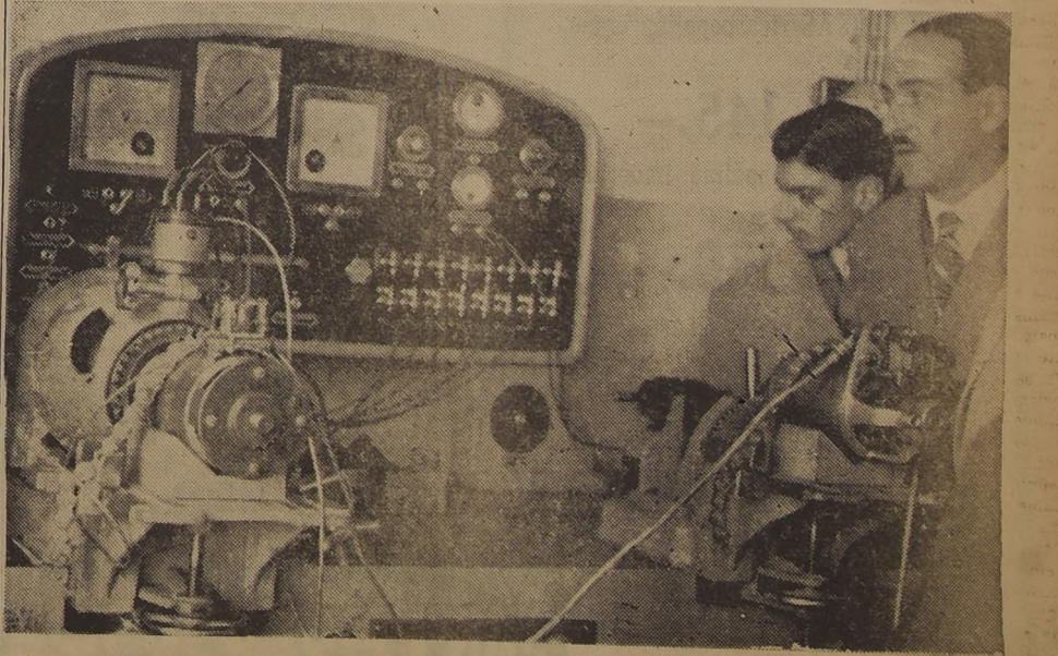
Máquina para probar todos los desperfectos eléctricos de los motores de los automóviles
