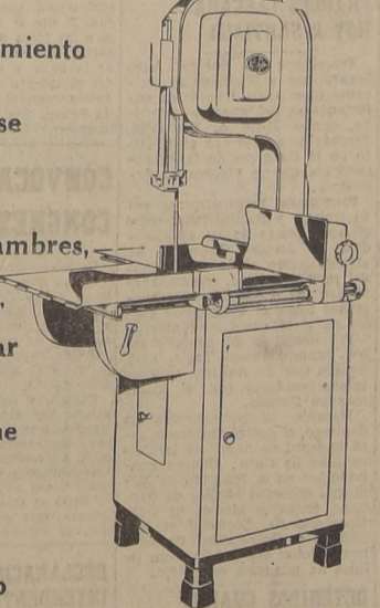
Sierra para huesos. — Para cortar huesos grandes y chicos sin astillarlos y con un corte finísimo.
