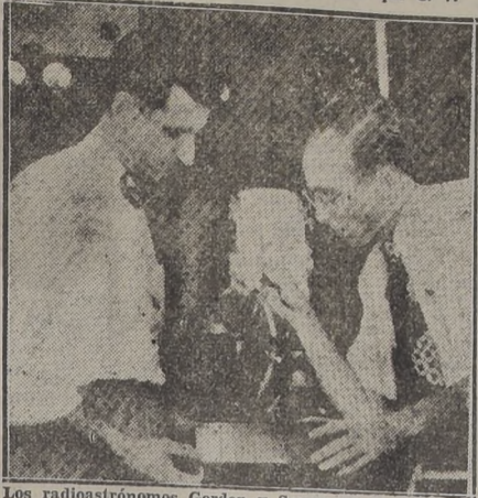
Los radioastrónomos Gordon y Seeger estableciendo el punto central de los ruidos de la Vía Láctea
