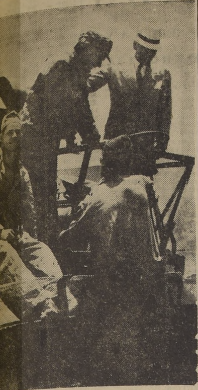
Los Servicios de Equipos Mecanizados de la Corporación de Fomento de la Producción, señor Alfonso Quintana Burgos, impone la reparación técnica de una trilladora. Le imponen el trabajo los señores Guillermo Zúñiga, Mario Becerra y José Rojas.
