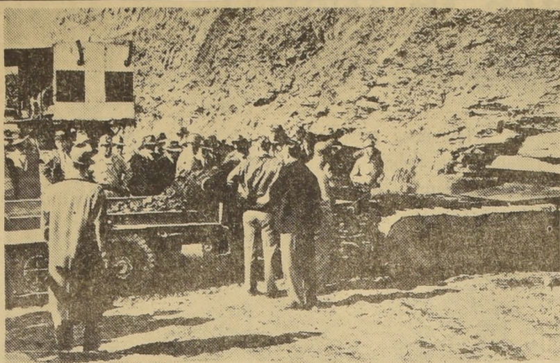
NEW LEXINGTON (Ohio). — El "Colmo", gigantesca máquina excavadora, que es capaz de extraer y cargar de 3 a 5 toneladas de carbón en un minuto. Se mueve hacia adelante bajo sus propios medios mecánicos, a la vez que extrae una apreciable cantidad de carbón, que es conducido por una faja de goma. Esta nueva y poderosa máquina para la minería fue construida por la Sunnyhill Coal Company (Foto ACME).
