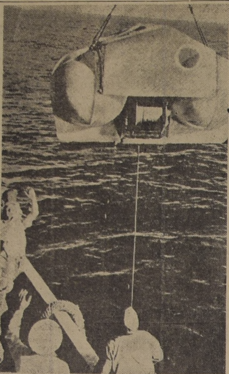
Esta complicada boya, provista de un cable de salvamento, ha sido ensayada con éxito en maniobras de rescate de submarinos, realizadas cerca de las costas inglesas.
