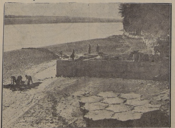
Una sección de aeródromo flotante, del tipo empleado en el Pacífico durante la guerra aparece en la foto en el instante en que es montado para establecer un puente provisional que, cruzando el río Severn, sirva al tránsito caminero entre las localidades de Newnham, en el lado galés de Gran Bretaña, y Arlingham, en el lado inglés. La faja de aterrizaje está compuesta por flotadores hexagonales, unidos por bisagras. (Foto BIPPA)
