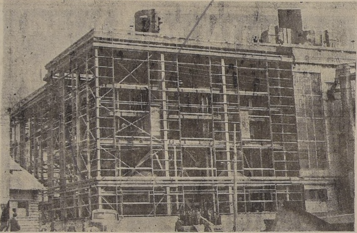
Una vista de la obra de ingeniería que se levanta junto a la antigua unidad de Laguna Verde. Tiene una altura de 27 metros, y es construida sólo de acero y cemento, capaz de resistir cualquier movimiento sísmico. Los trabajos son realizados por ingenieros, técnicos y obreros chilenos, bajo la supervigilancia de peritos norteamericanos.
