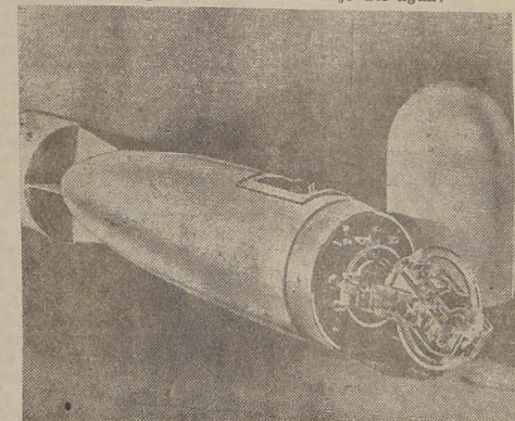
La búsqueda de petróleo debajo del mar puede efectuarse desde el aire. Ella se realiza mediante inspecciones magnéticas hechas con un magnetómetro —como el que aparece en la fotografía—, que cuelga de un avión
