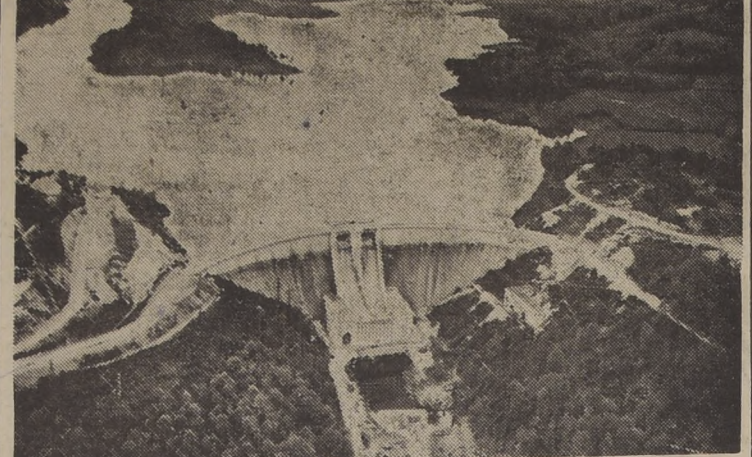
Entre las grandes obras de ingeniería que se han realizado últimamente en Francia, es digno de señalar la gigantesca represa de Saint Etienne, que nos muestra esta hermosa fotografía.
