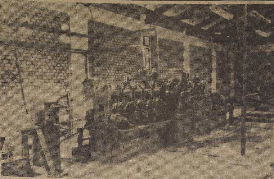
La máquina en que se fabrican los tubos de acero en pleno funcionamiento.
