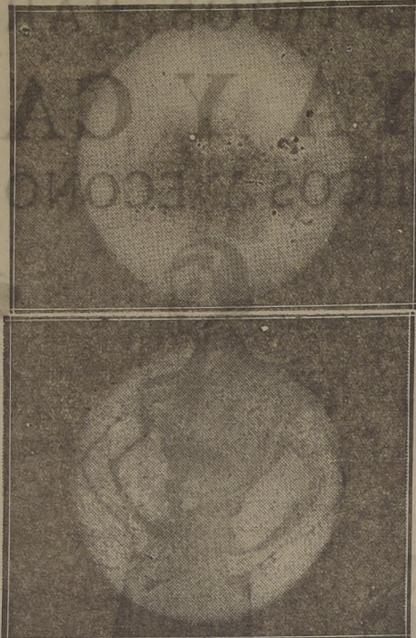
Dos aspectos del Sol: la figura superior presenta la fotosfera con sus manchas, y la figura inferior, la cromosfera con los filamentos de hidrógeno. Dentro de 300 años, las fuentes actuales de energía: carbón, gas y petróleo, se habrán agotado, y entonces será necesario recurrir a la energía solar.
