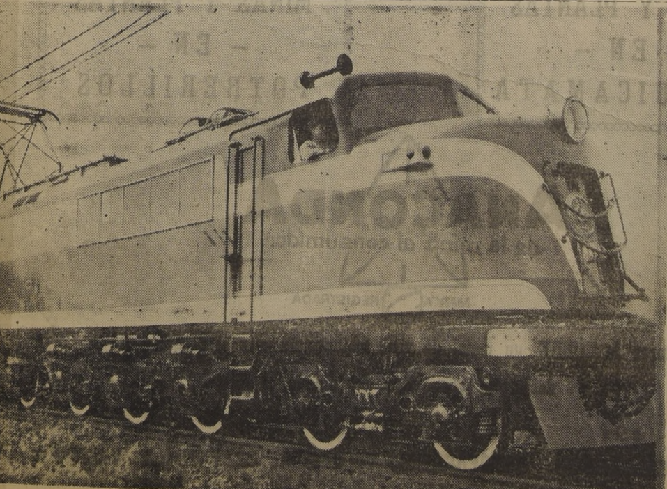
Aspecto de la locomotora de la General Electric, poderosa unidad de 210 toneladas de peso y de una potencia de 4.000 HP., que ha sido puesta en servicio entre Valparaíso y Santiago
