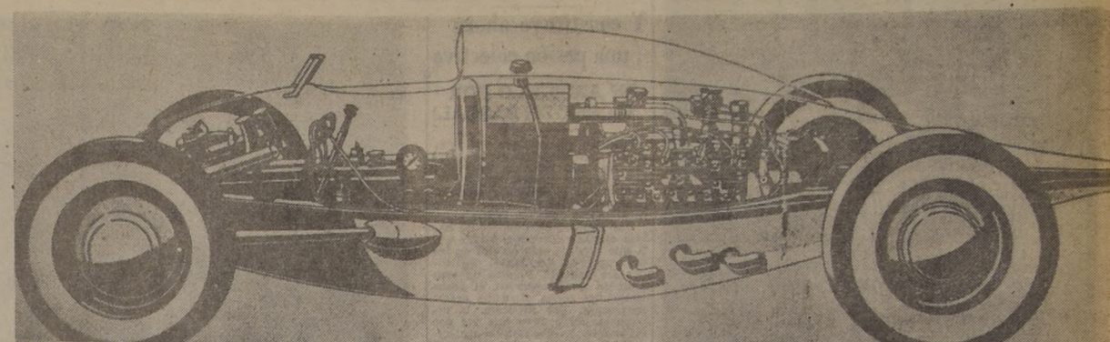
CON EL MOTOR ATRAS Y SIN RADIADOR. — Ni tampoco tiene caja de velocidades. Todo esto se ha hecho para ahorrar peso. Este es el diseño del "hot rod", mezcla de chasis "T" y "A" de Ford V-8. Con él han logrado, los "líricos" de California, la extraordinaria velocidad de 243.095 kilómetros por hora.
