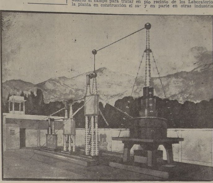
Perspectiva del lado interior de la instalación desintegradora.
