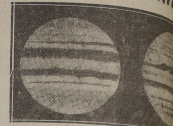
Dos dibujos de Júpiter, en los que se ve el planeta del mismo, de un satélite y sus órbitas.
