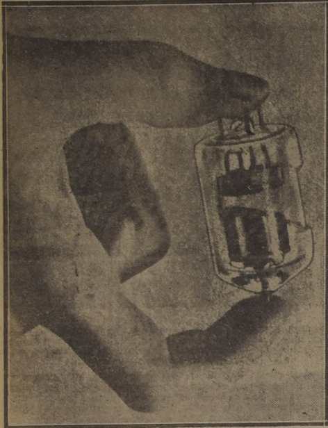
LAMPARA DE RAYOS X que se considera la más pequeña que se haya fabricado. Ha sido diseñada especialmente para trabajos dentales; tiene una producción de radiación concentrada y estabilizada, lo que provoca alto contraste y gran precisión en la placa que se obtiene
