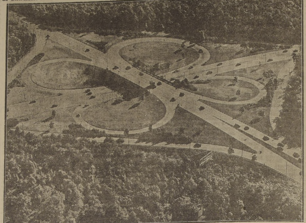
La congestión del tránsito es otro de los problemas que se agravarán en el correr del tiempo, ya que aumentarán la población y los vehículos. La fotografía muestra dos importantes arterias cerca de Nueva York, conectadas en forma de trébol de cuatro hojas, para evitar las aglomeraciones y los accidentes del tránsito.
