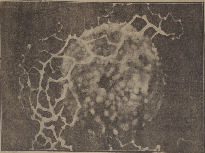
Ciertas sustancias predisponen al cáncer. Los químicos muestran ejemplos de su localización en los átomos.
