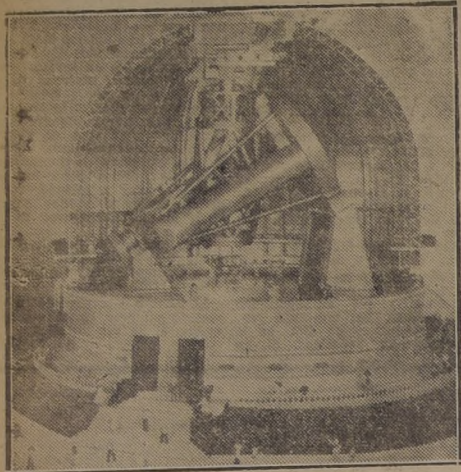
El famoso telescopio de Monte Palomar, en California, a pesar de ser el más gigantesco que se ha construido hasta la fecha, no es adecuado para el tipo de investigación que se propone realizar el Dr. Bok.
