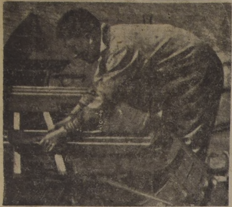
Aquí vemos trabajando en la colocación y ajuste de los carros al mecánico MANUEL HENRÍQUEZ, que ha resultado un experto en la construcción de estos accesorios de los botes de carrera. Los remeros de Talcahuano utilizarán estas embarcaciones en las regatas del 14 y 15 de octubre, con motivo de la celebración del IV Centenario de Concepción, torneo que está levantando enorme entusiasmo en todos los círculos.
