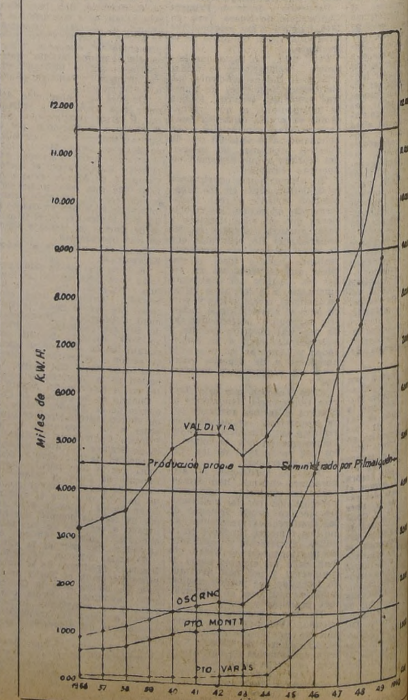
Gráfico que muestra el desarrollo alcanzado en los consumos eléctricos de las ciudades de Valdivia, Osorno, Pto. Montt y Pto. Varas, desde su conexión en 1944, al sistema Pilmaiquén.
