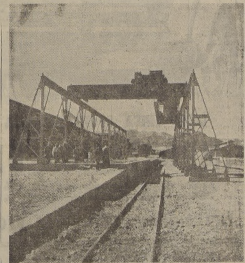
Puente grúa para descarga de minerales. Estos llegarán en carros de ferrocarril, por un desvío de 2,7 kilómetros, ya terminado y en servicio.
