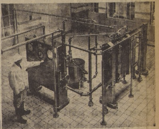
ESTA ES UNA PLANTA PASTEURIZADORA construida por la A.P.V. Es del mismo tipo de la que ha adquirido la SOPROLE S. A. — El lector puede observar los tubos e instrumentos de control y limpieza. El personal que trabaja en ella es muy limitado, y ninguna persona interviene, con la producción, una vez que ha sido vaciada la leche a los estanques. Después de un perfecto sistema de pasteurización, al final del proceso, la leche sale embotellada y lacrada para el consumo popular.
