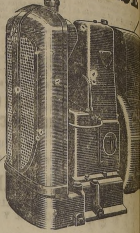
El Diesel Fairbanks-Morse de 5 1/4 H.P. es un motor vertical, monocilíndrico, de cuatro tiempos, de fuerte y sólida construcción, con lubricación por presión.
