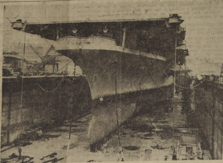
El "Tarawa" de la Flota de Reserva de los Estados Unidos puesto en servicio activo. Con este barco ya suman 165 puestos en servicio por la Reserva del Atlántico de aquel país. El transporte tiene una tripulación normal de 2.500 oficiales y hombres, puede transportar cuatro escuadrones de aviones, o sea un total de 75 a 100 unidades, según el tipo.
