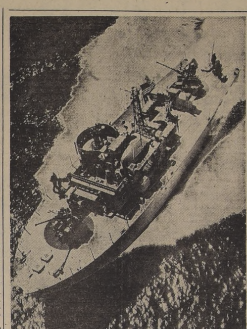
Construido de aluminio, un nuevo patrulla-torpedo de la Marina de los Estados Unidos, tiene su estructura en parte soldada a soplete y en otras remachada. El PT-810 es una de las embarcaciones más rápidas y más livianas con que cuenta la Marina de los Estados Unidos de América. En esta foto vemos a una de ellas maniobrando en la bahía de Chesapeake, a la salida de Baltimore en el Estado de Maryland. — (USIS).
