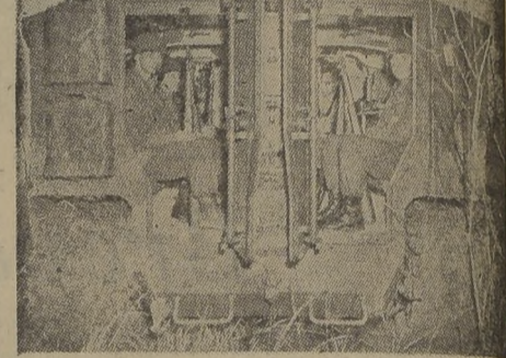
CARRO BLINDADO PARA EL TRANSPORTE DE INFANTERÍA: vista exterior (Arriba), e interior (Abajo), del nuevo transporte adoptado por el ejército norteamericano para proteger a las tropas en camino al frente de batalla, de los tiros de fusiles, ametralladoras y cascos de granadas. Tienen capacidad para transportar 12 soldados, y pesan 20 toneladas. Pueden ser empleados asimismo para transportar municiones, como carro del comandante en el campo de batalla o como ambulancias.—("The Sphere", Londres).
