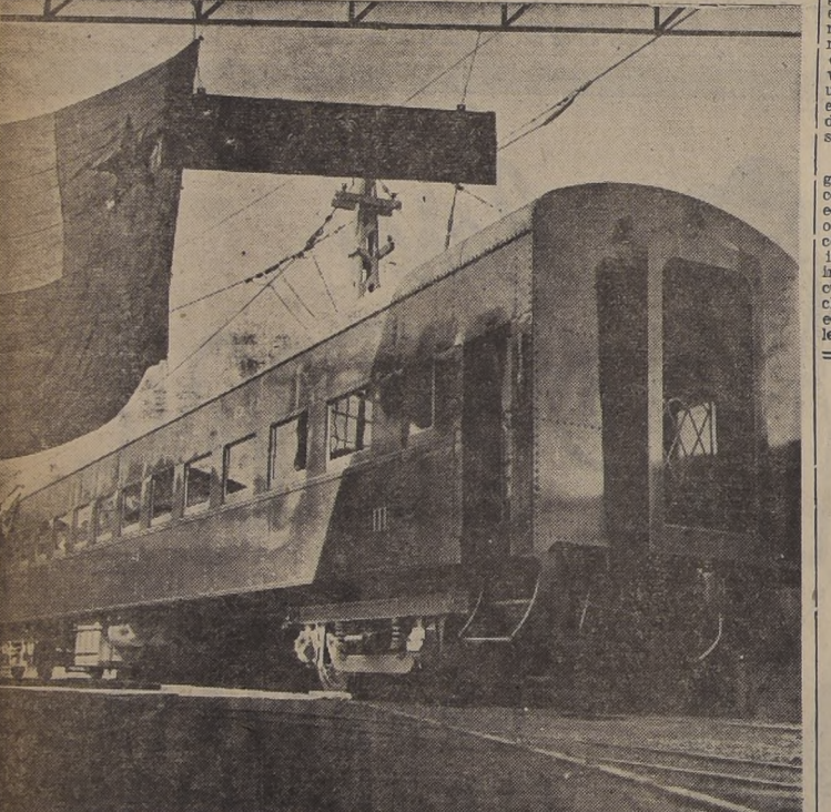
Vista exterior del nuevo coche de pasajeros para tercera clase, totalmente de acero, construido en los talleres de Socometal. El vagón posee aislación térmica de lana de vidrio y todas las características de seguridad de los coches de lujo
