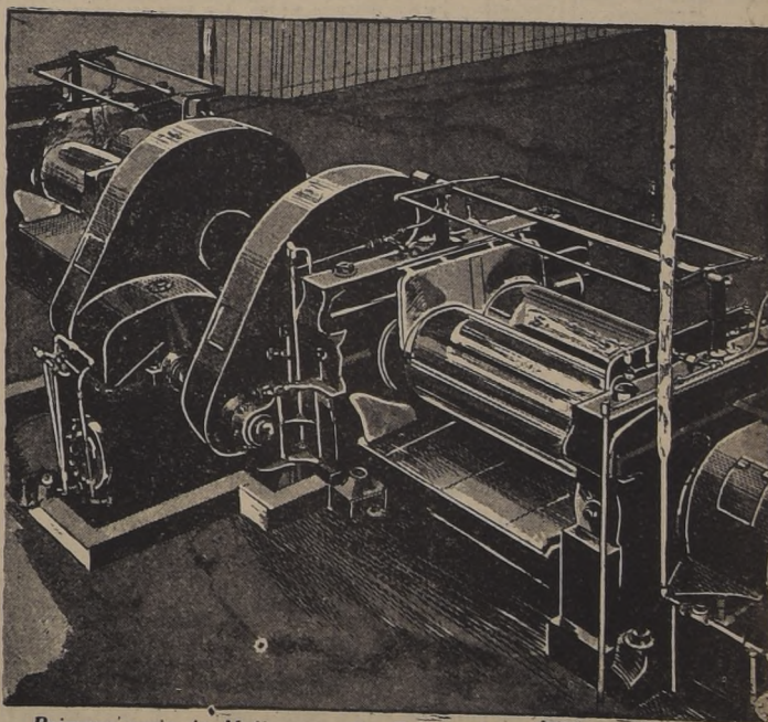
Primera serie de Molinos a alta Temperatura, donde se inicia el proceso automático para elaboración de los Plásticos Flexibles de IMPLATEX
