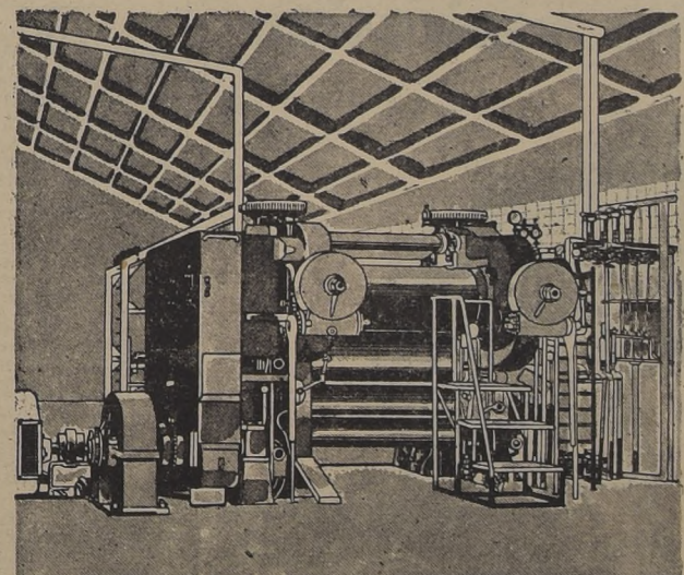
Aspecto parcial de la Calandria gigante, empleada en uno de los procesos de elaboración de Plásticos Flexibles. Es la única de este tipo montada en Sud-América
