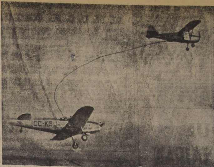
ABASTECIENDO EN VUELO. — En el grabado vemos el momento en que el avión Cesna ha tomado contacto con el Fairchild que lo abastecerá por medio de una manguera de nylon, de media pulgada.
