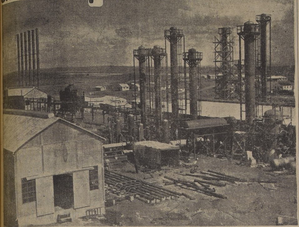
Ciento cincuenta obreros especializados, que se formaron técnicamente en los propios yacimientos de Cerro Manantiales, levantan la primera refinería que producirá gasolina chilena.—El grabado muestra las dos secciones de esta planta cuyo rendimiento será de 47 mil 900 litros diarios de gasolina, además de una gran cantidad de subproductos.—Esta refinería entrará en funciones en abril próximo
