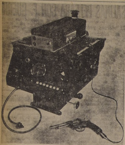
EL RACEND OMEGA TIMER. — Este es el más complejo de los aparatos que se utilizarán para cronometrar los diferentes deportes en Helsinki.
