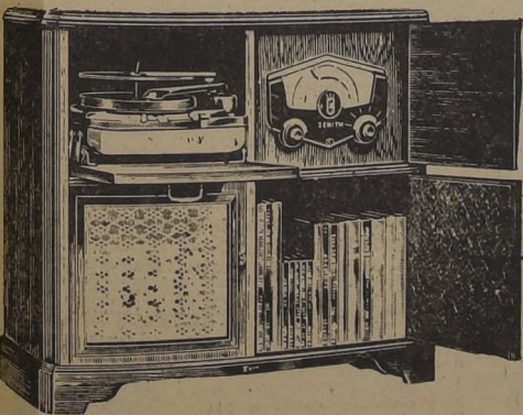
Mod. J 518 Onda corta y larga, corriente universal. Gran potencia de salida.
